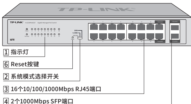
图1-4 YLS220P-16G2F前面板示意图
