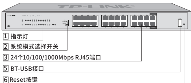
图1-3 YLS220MP-24G前面板示意图
