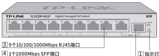
图1-5 YLS220P-9G1F前面板示意图
