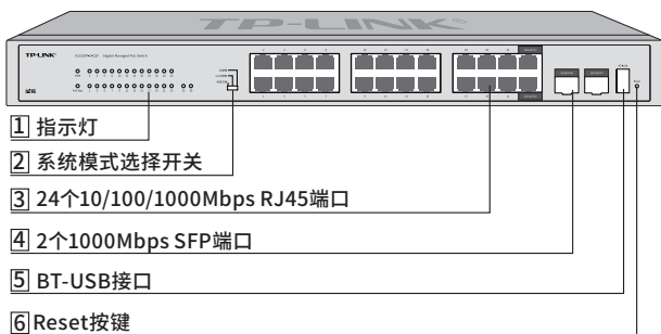
图1-2 YLS220P-24G2F前面板示意图
